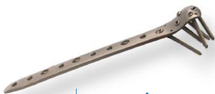
PLACA FÊMUR PROXIMAL LATERAL 4.5MM
